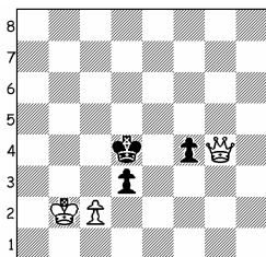
H # 2 zero a) +♜e5, b) +♜c6
