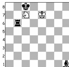
H # 3 zero a) ♜>b7, b) ♜>h2
