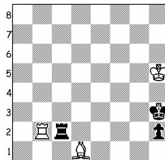
H # 2 2.1... b) ♖>e2
